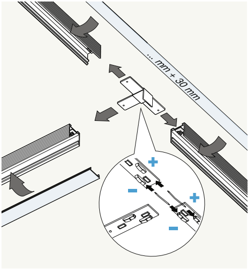
XM2033-UT Giunzione T trimless T junction trimless
