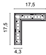
0971 Angolo 90° - 90° corner .01 Bianco - White
