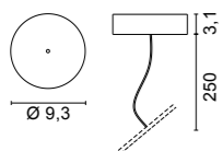
0946 Rosone completo di cavo di alimentazione. Ceiling rose with cable. .01 Bianco - White
