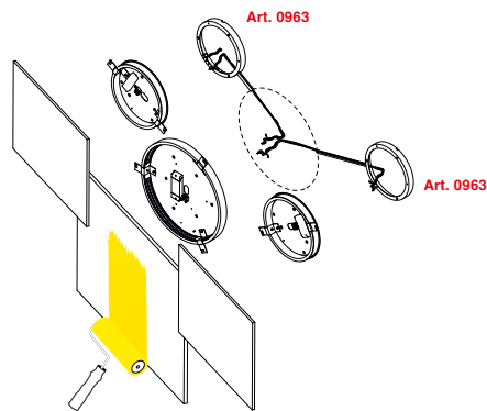
Esempio di installazione multipla con distanziali. Example of multiple installation with spacers.
