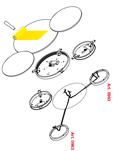
Esempio di installazione multipla con distanziali. Example of multiple installation with spacers.
