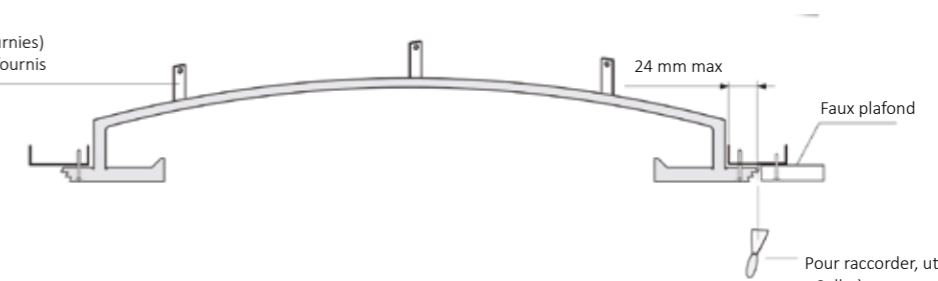
Schéma de pose d'une coupole encastrée
